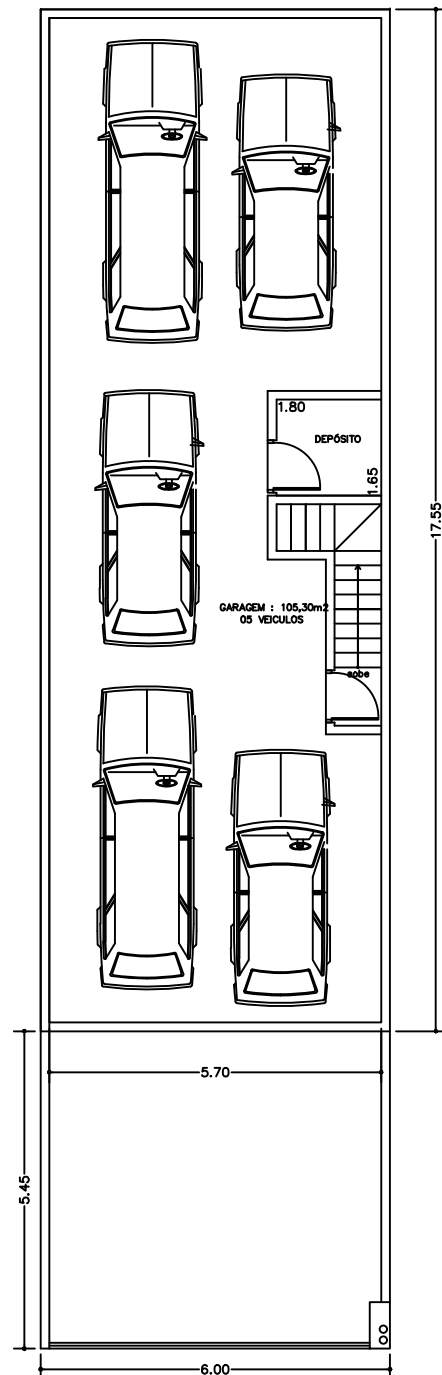
Planta Baixa - Pav. Inferior PAV. INFERIOR = 105.00 M 2 ÁREA TOTAL CONSTRUÍDA = 255.00 M 2
