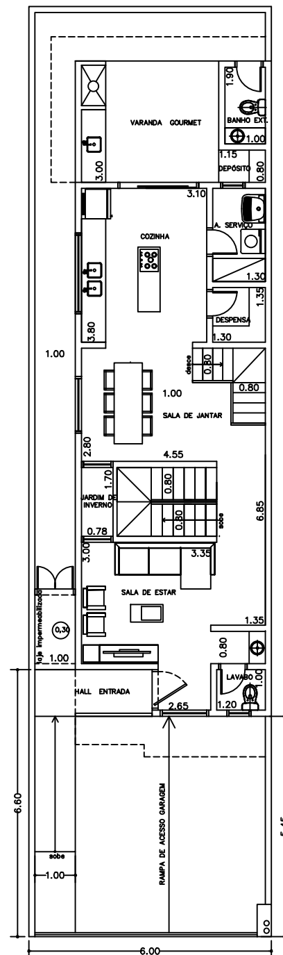
Planta Baixa - Térreo PAV. TÉRREO = 81.70 M 2 ÁREA TOTAL CONSTRUÍDA = 255.00 M 2
