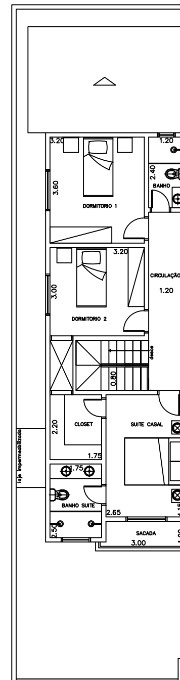
Planta Baixa - Pav. Superior PAV. SUPERIOR = 68.30 M 2 ÁREA TOTAL CONSTRUÍDA = 255.00 M 2
