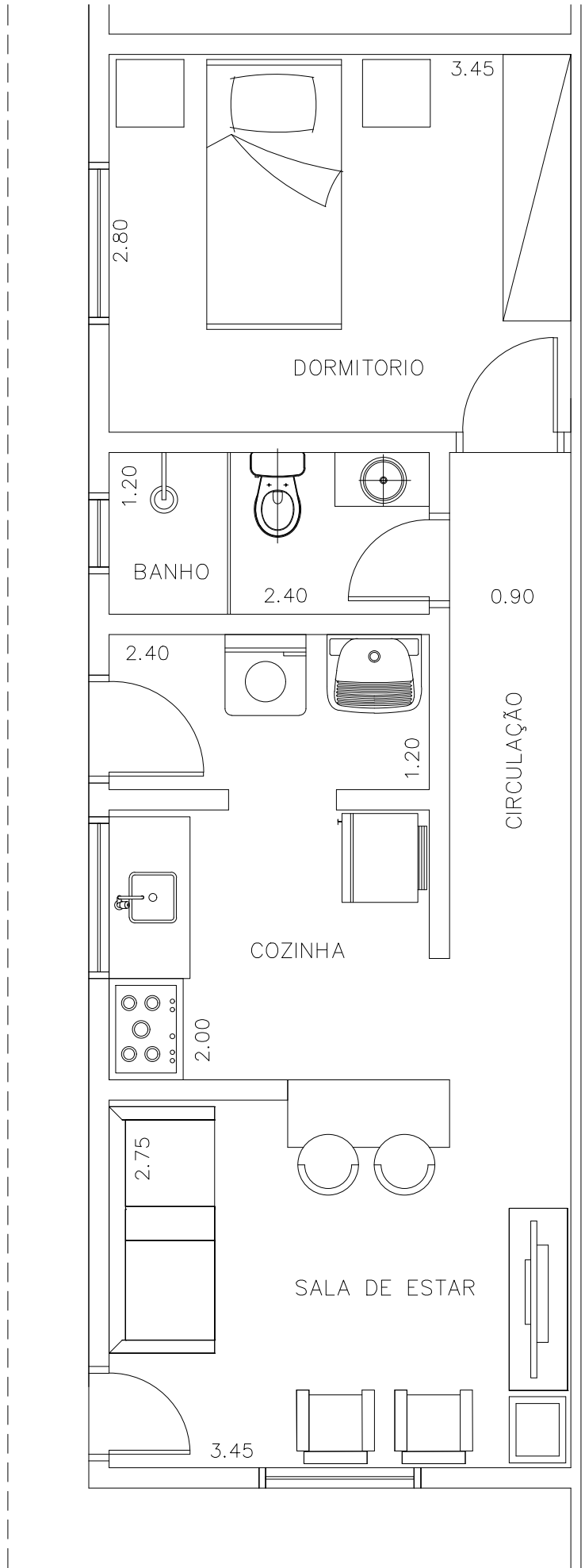
Planta Baixa – Unidade Padrão ÁREA TOTAL CONSTRUÍDA = 39.05 M2
