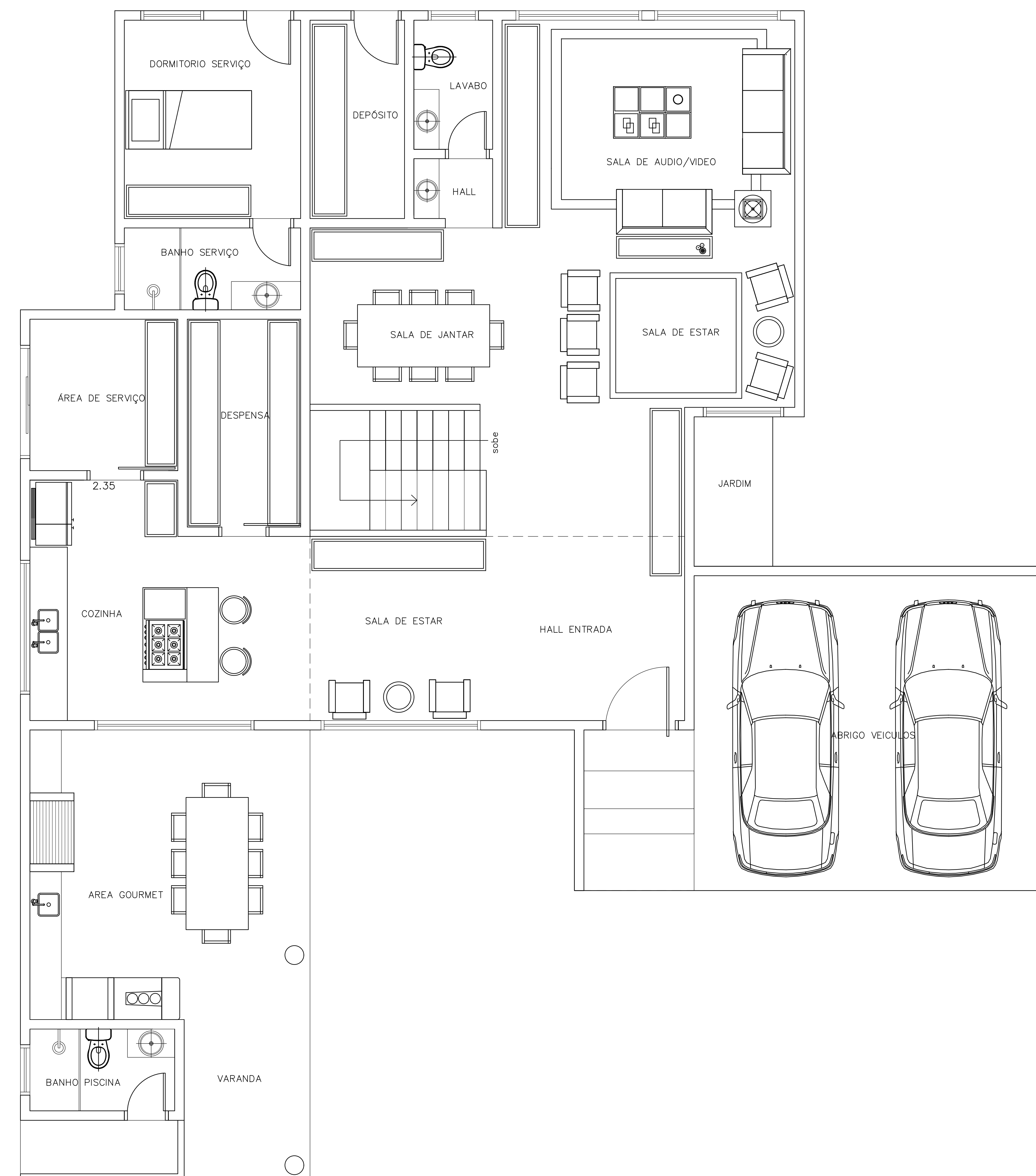
Planta do pav. terreo ÁREA CONSTRUÍDA PAV. TERREO = 193.20 M2
