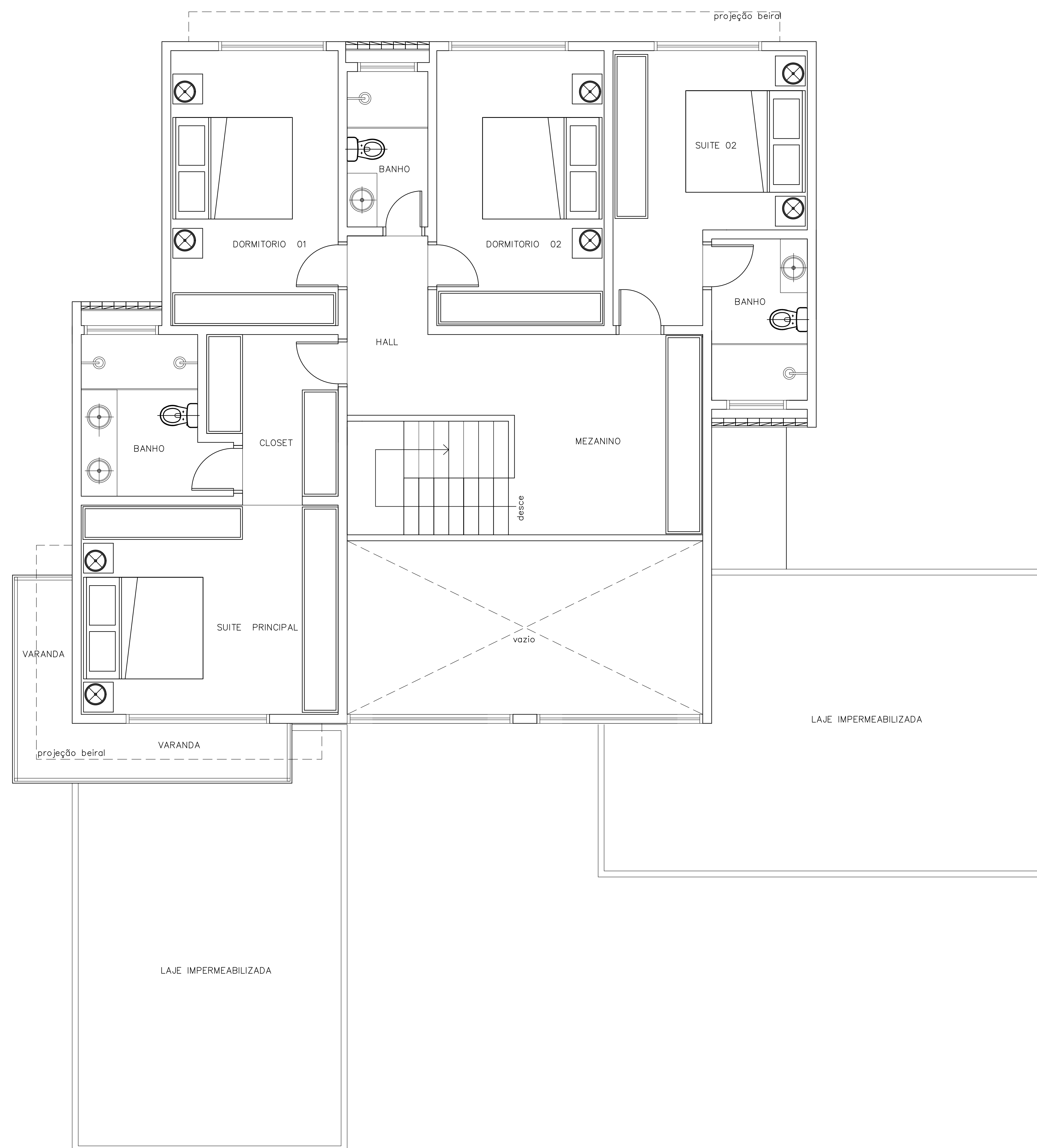
Planta do pav. superior ÁREA CONSTRUÍDA PAV. SUPERIOR = 109.70 M2
